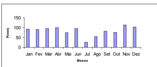
Figura 5 - Quantidade de Precipitação Máxima Diária
