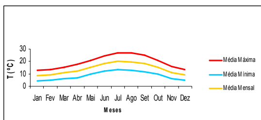
Figura 2 - Temperatura Média Mensal
